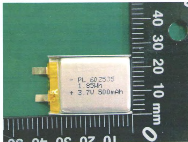
元件电池 Component Cell
