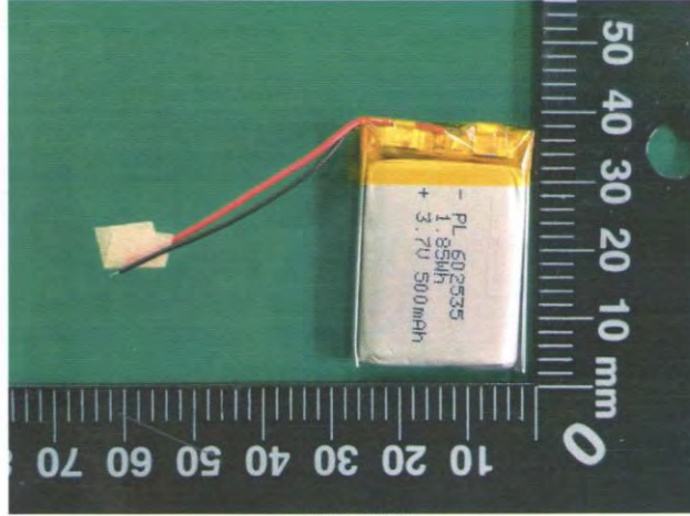
电池组 (正面) Battery (top view)
