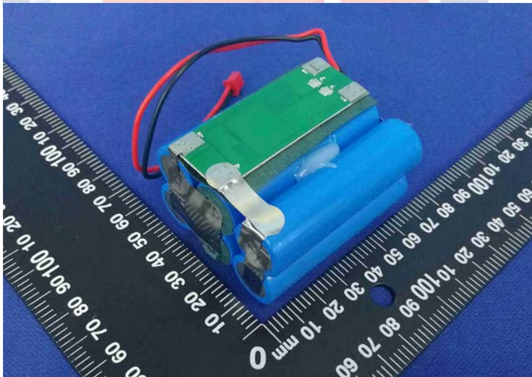
Picture 4. Back view of cell 图片 4. 电池后视图
