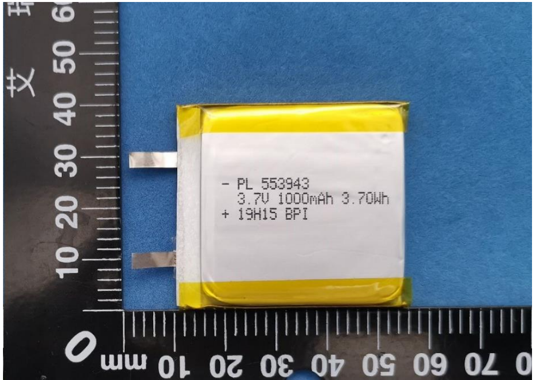
Cell /电芯 (PL 553943 3.7V 1000mAh 3.7Wh)
